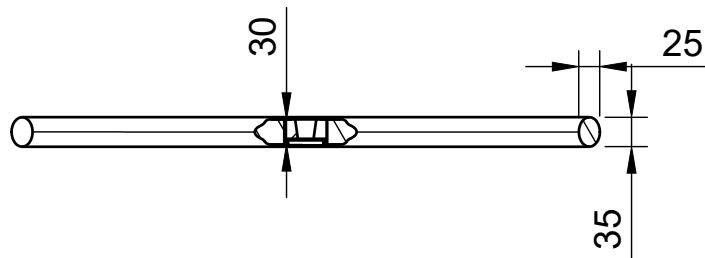
A-A (1:9)
