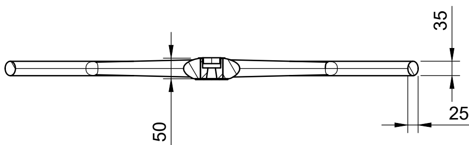
A-A (1:9)
